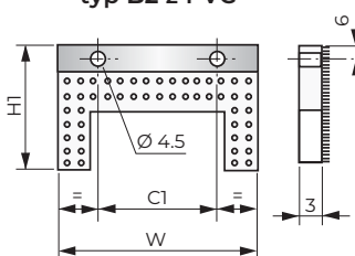
standardní příruba typ B2 z PVC
