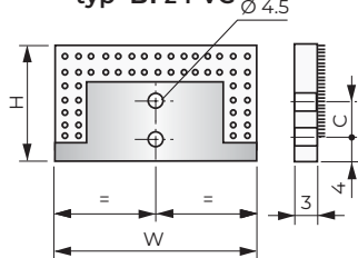
standardní příruba typ B1 z PVC
