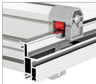
Guia de travessa
