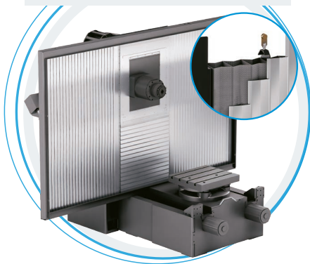
KRYTOVACÍ SYSTÉMY X-Y S OCHRANNÝMI MĚCHY X-Y SHIELDS WITH BELLOWS
