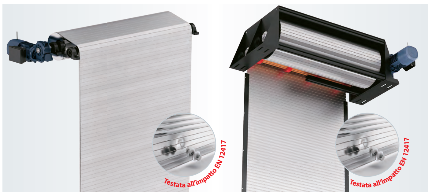
VERSIONE SENZA CASSONETTO E CON RULLO DI RINVIO DELLA TAPPARELLA
