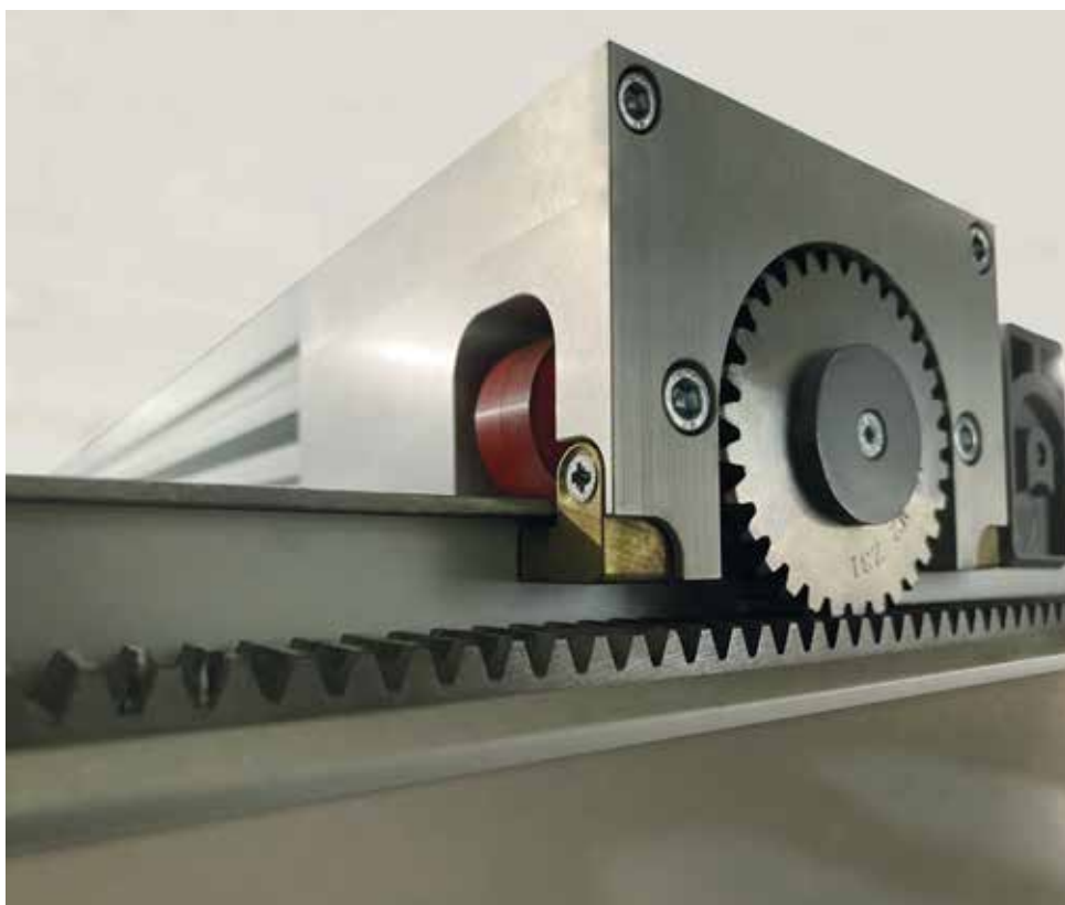
Smart Drive HP: la nuova motorizzazione della linea Wave Sky, protezione per la protezione del cielo di fresatrici a traversa mobile ( https://www.pei.it/it/prodotti/soffietti-di-protezione-per-cieli-wave-sky/ ).
